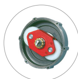
Планетарный редуктор (L16)
