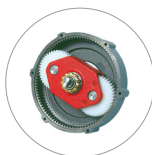
Engranaje planetario
