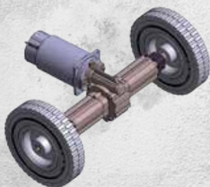
Motodifferenziale
